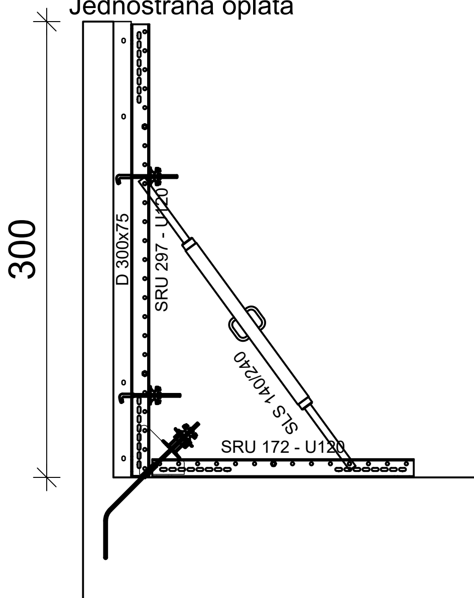
KARAKTERISTICAN PRESEK Jednostrana oplata
