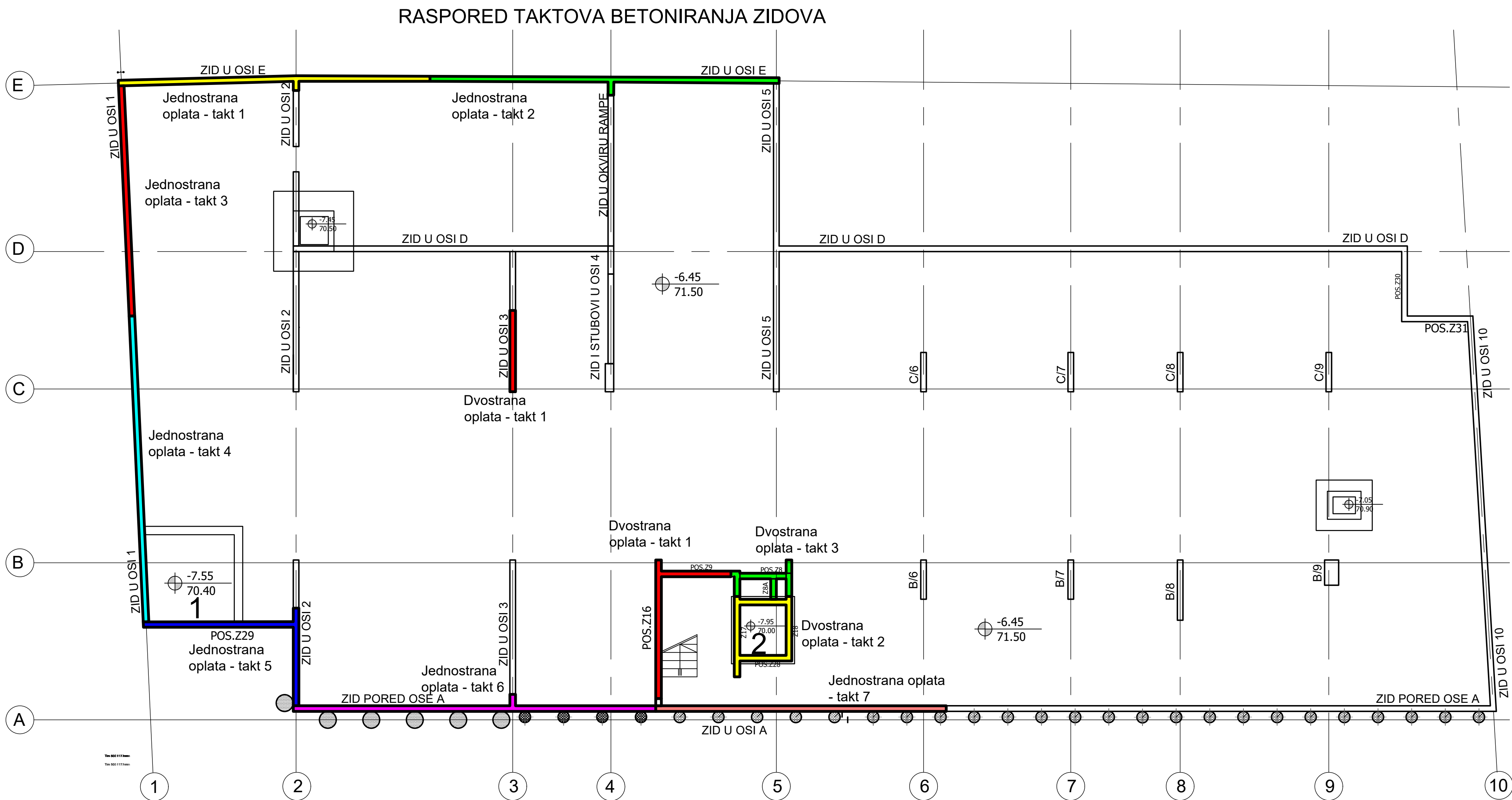
JEDNOSTRANA OPLATA - ZID U OSI A - TAKT 6
