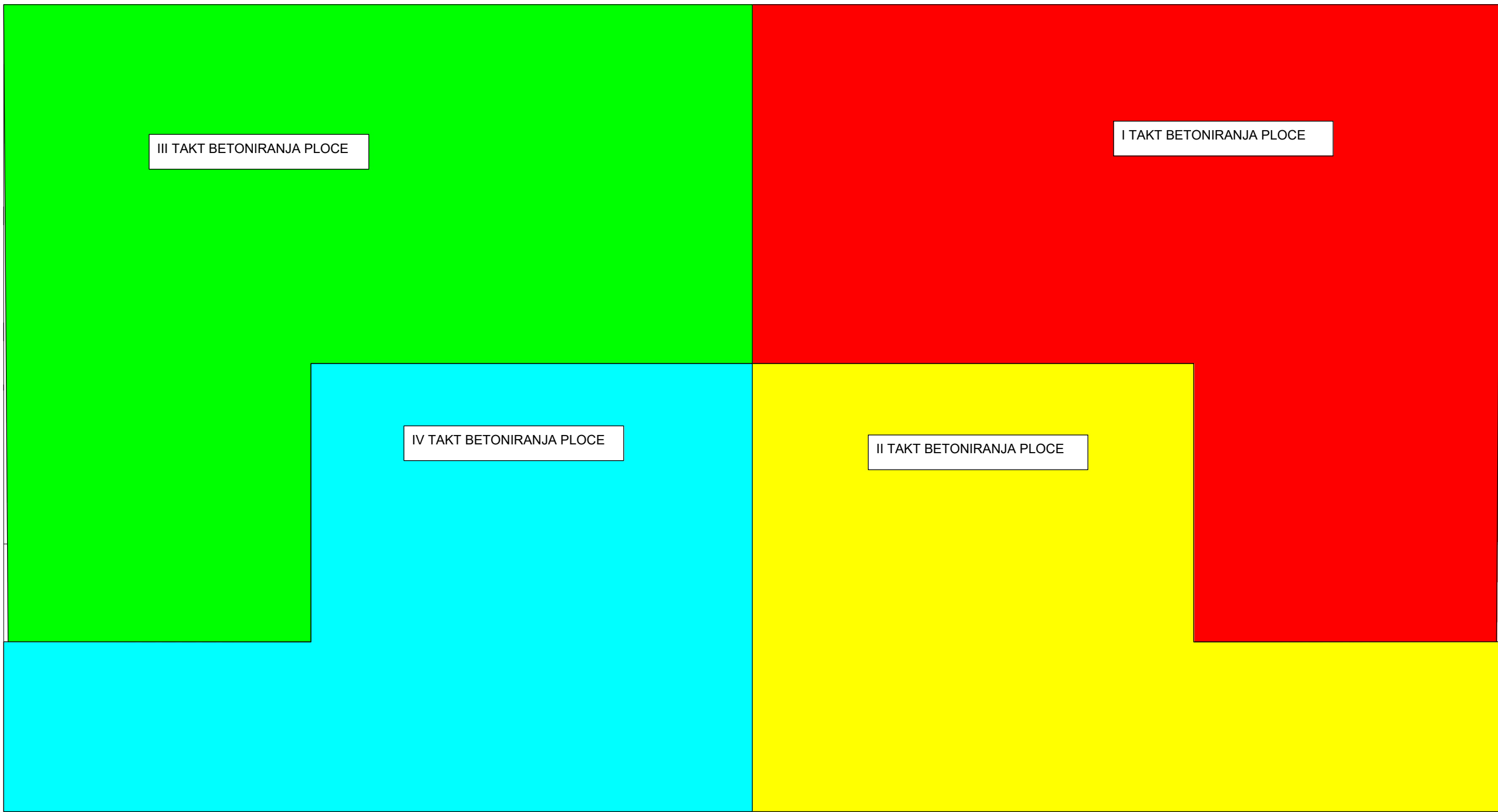
PREDLOG TAKTOVA BETONIRANJA PLOCE PODRUMA
