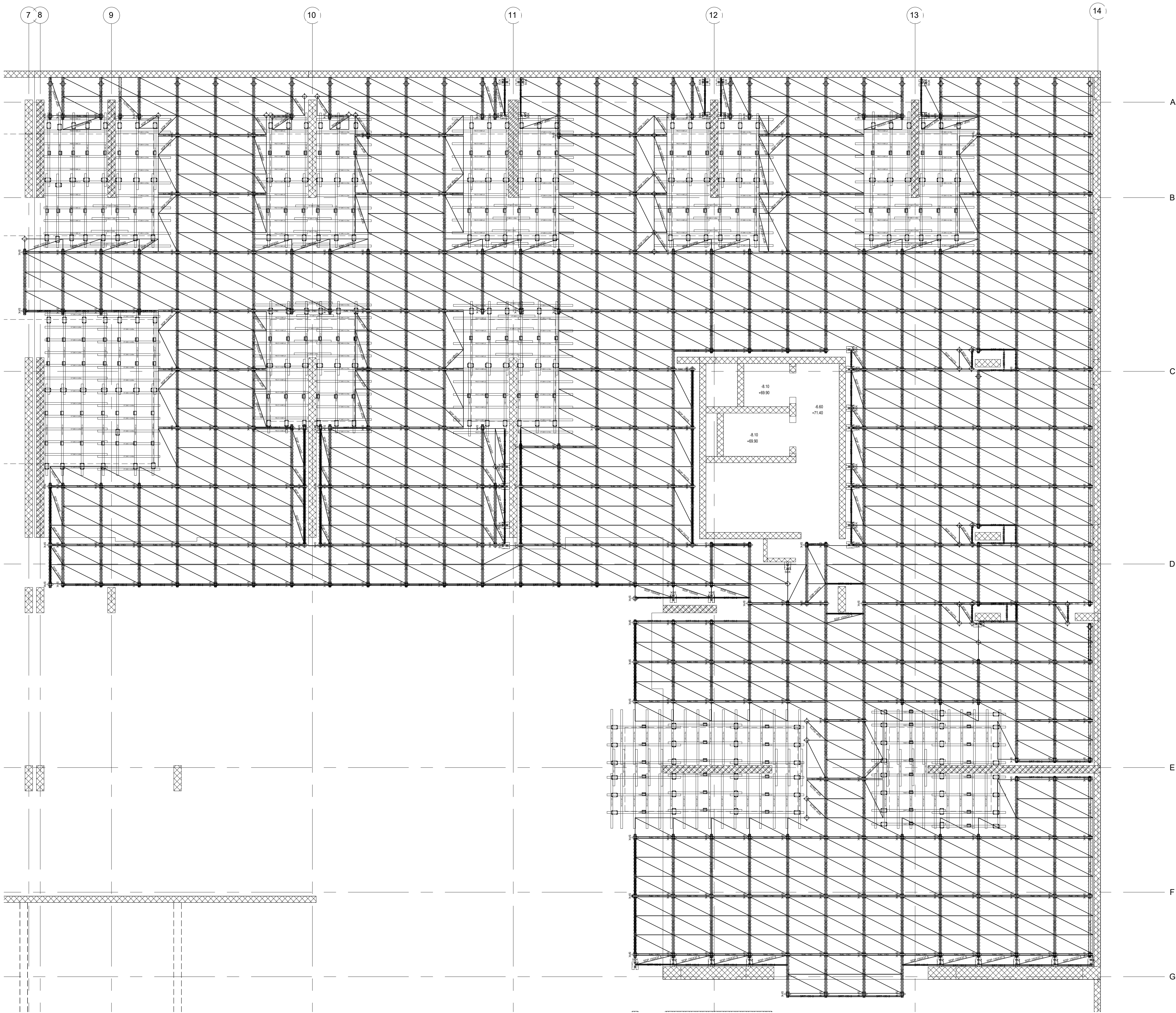
PLAN OPLATE PLOCE PODRUMA - I TAKT BETONIRANJA
