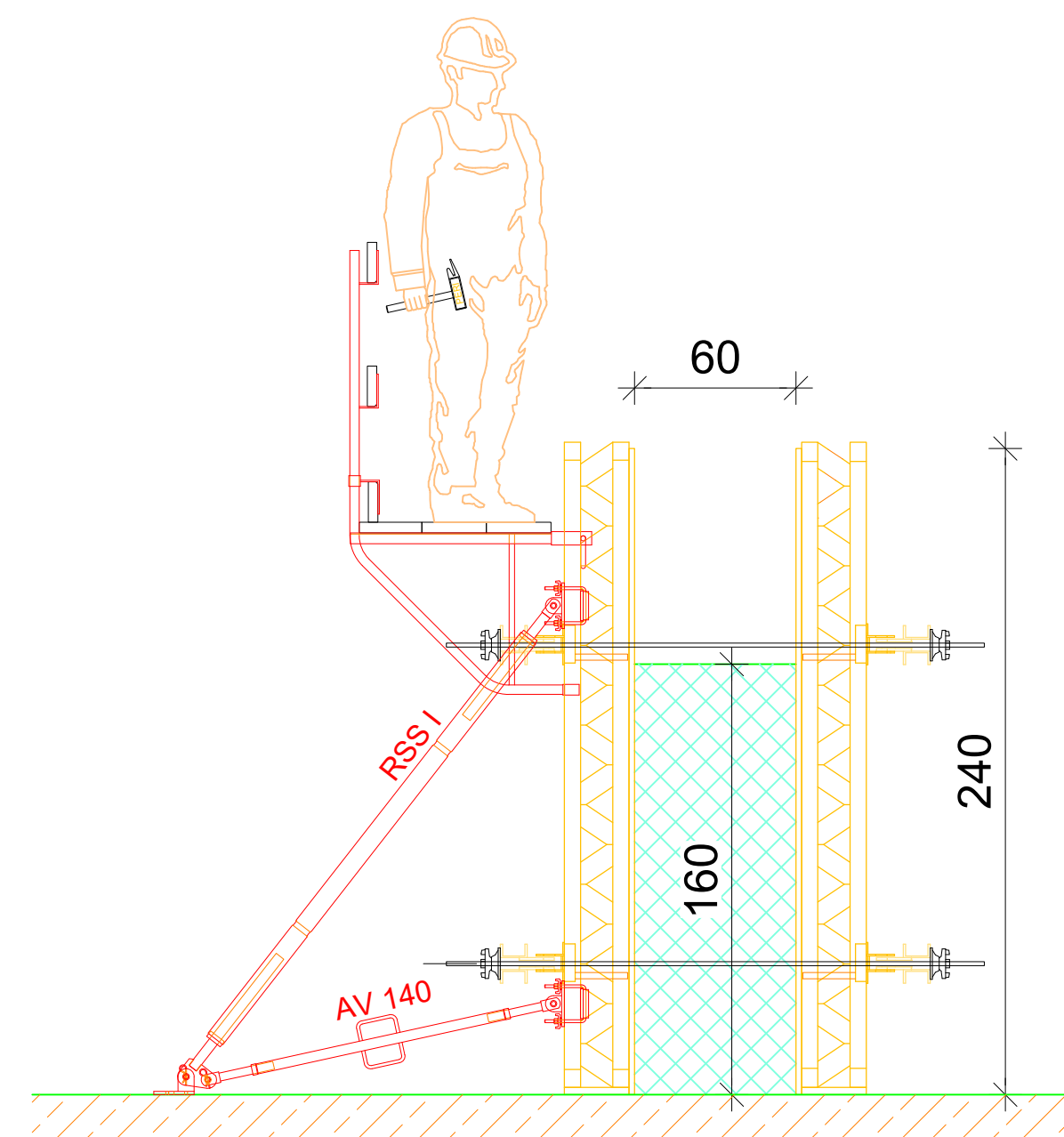
Karakteristični poprečni presek
