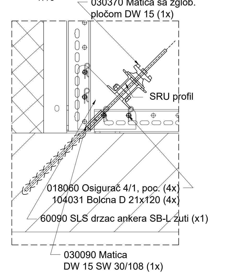
Detalj ankerisanja 1:10
