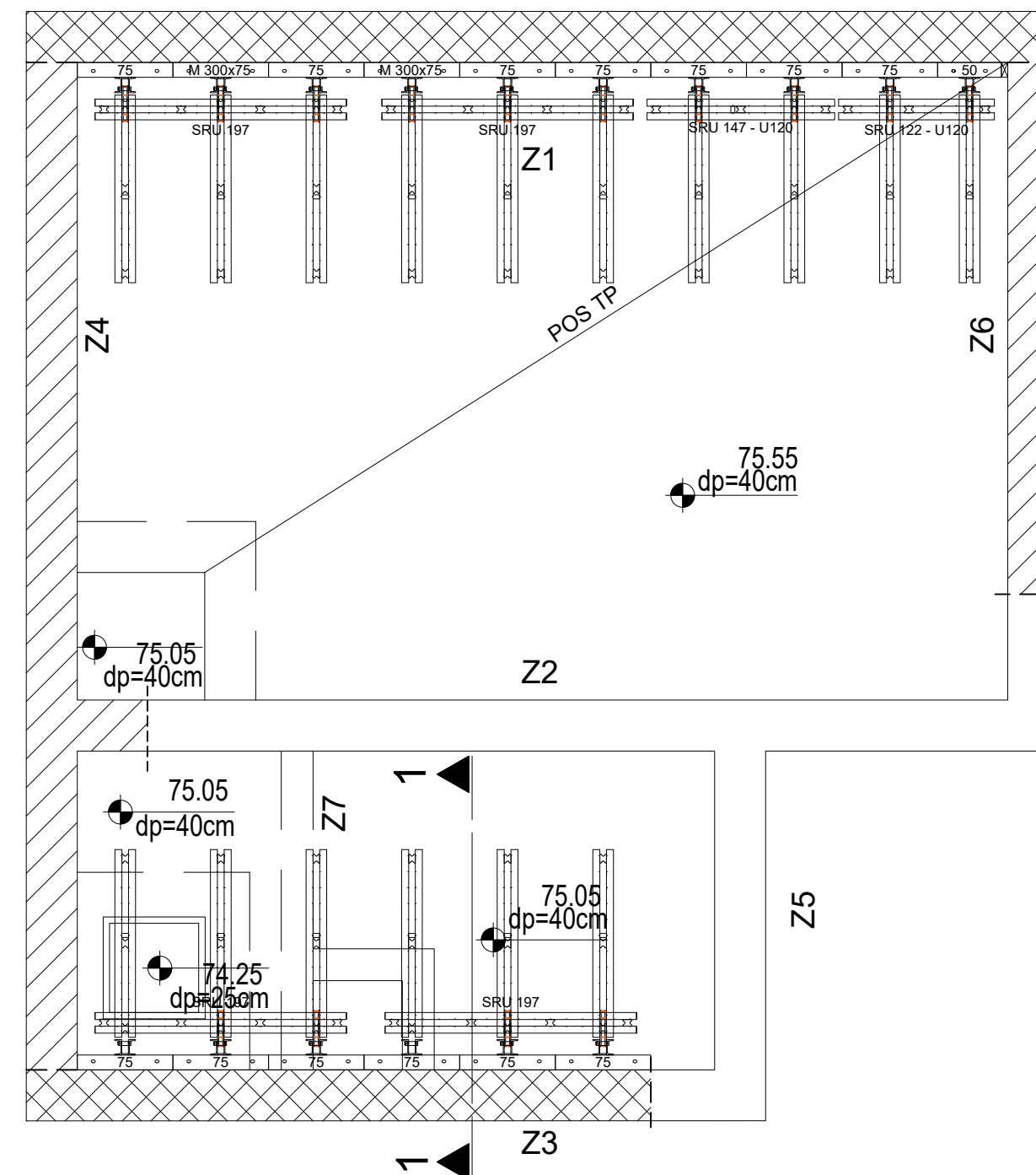
Osnova TAKT 03 - dvostrana oplata
