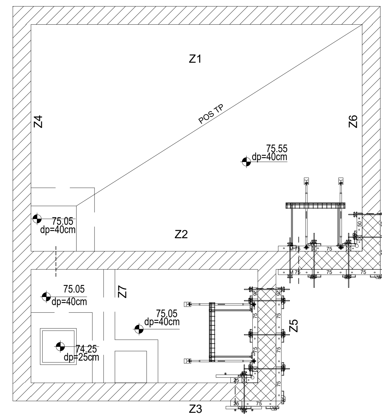
Osnova TAKT 04 - dvostrana oplata 1:50
