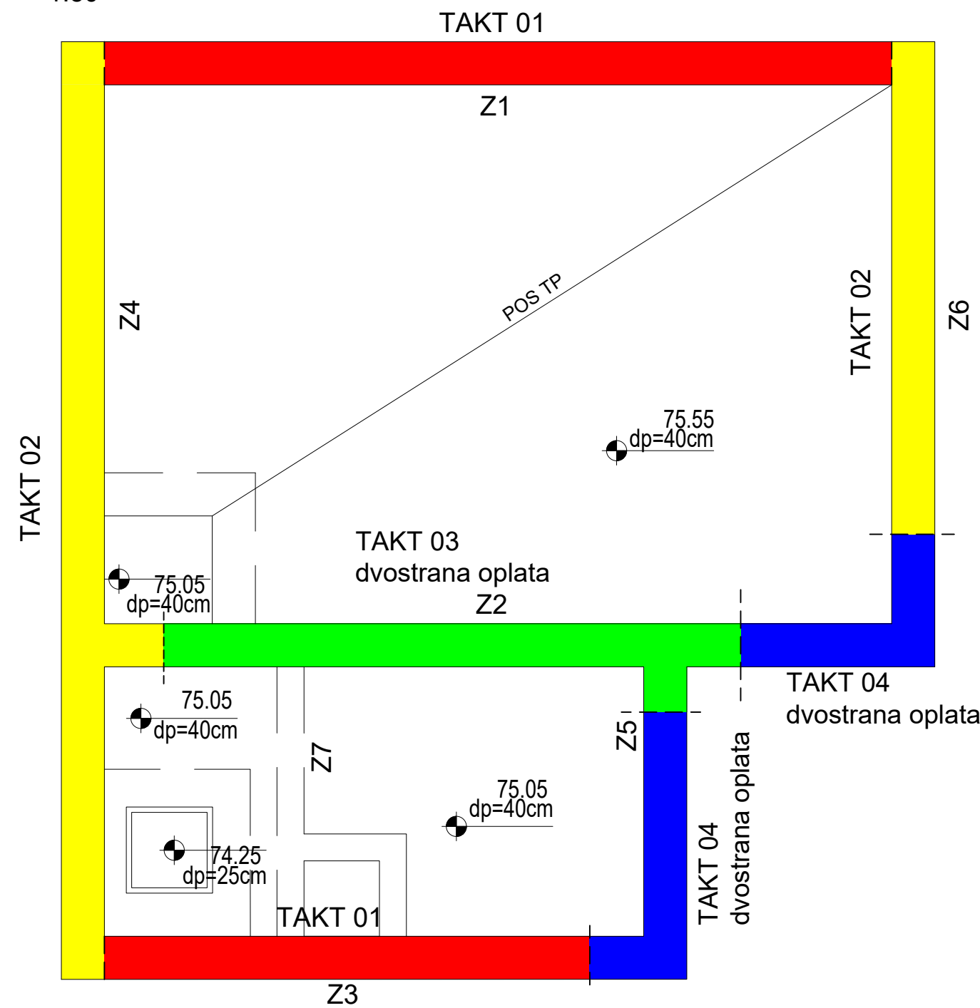
Osnova raspored taktova
