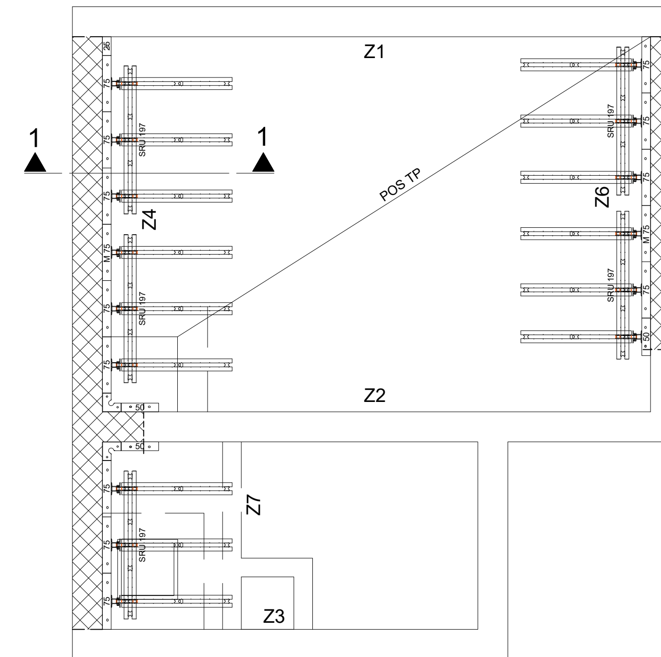
Osnova TAKT 02 1:50
