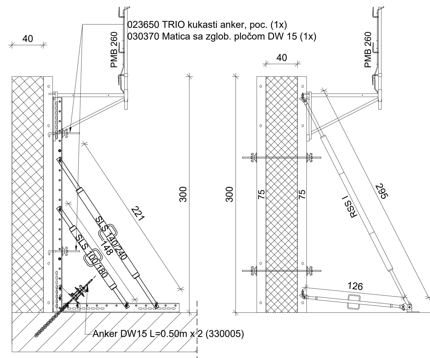
Presek 1-1 1:25
